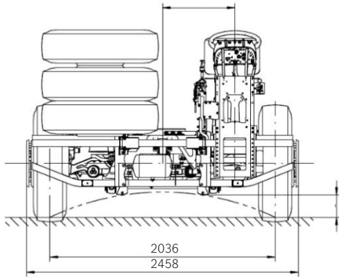
Tampak Depan
