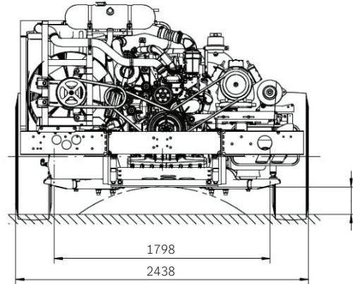
Tampak Belakang
